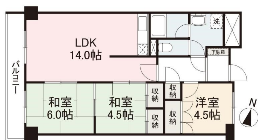
【間取り図】
